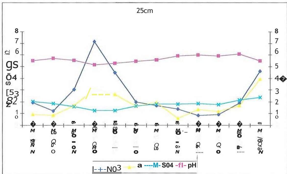
Figura 25 - Concentração de cátions (C \blacklozenge K, Na) e ânions (N-NO 3 , Cl, S-SO 4 ) e pH, na solução do solo, na profundidade de 25 cm, no estudo de Klinge (1998).
