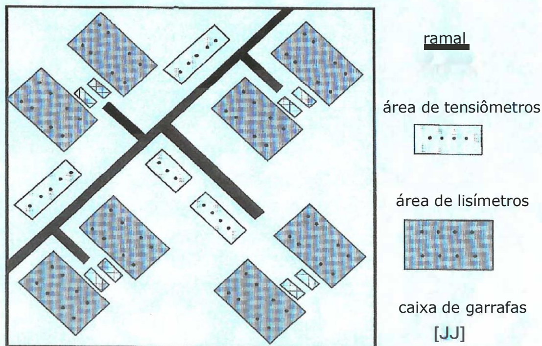
Figura 10 - Esquema geral das instalações dos lisímetros.
